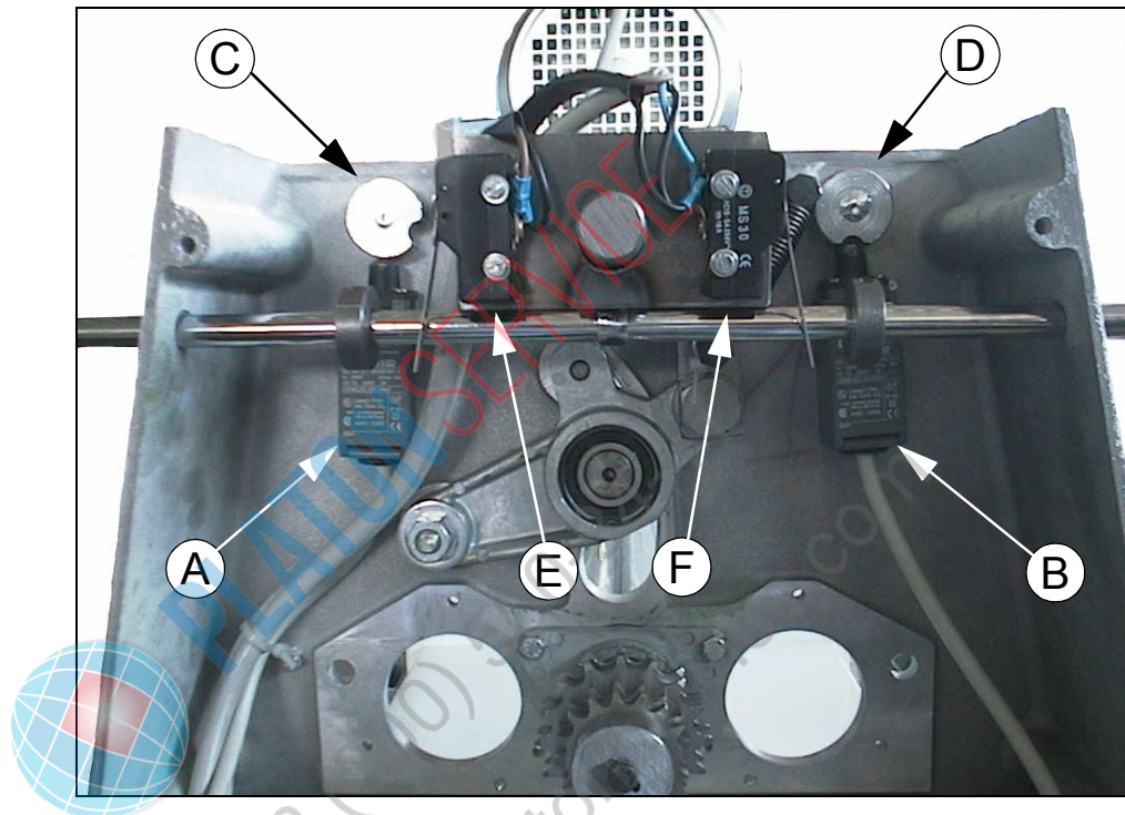
Fig. 1.3 Microswitch
